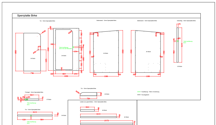
Abbildung 7: Ausschitt CNC Plan Quelle: öKlo
