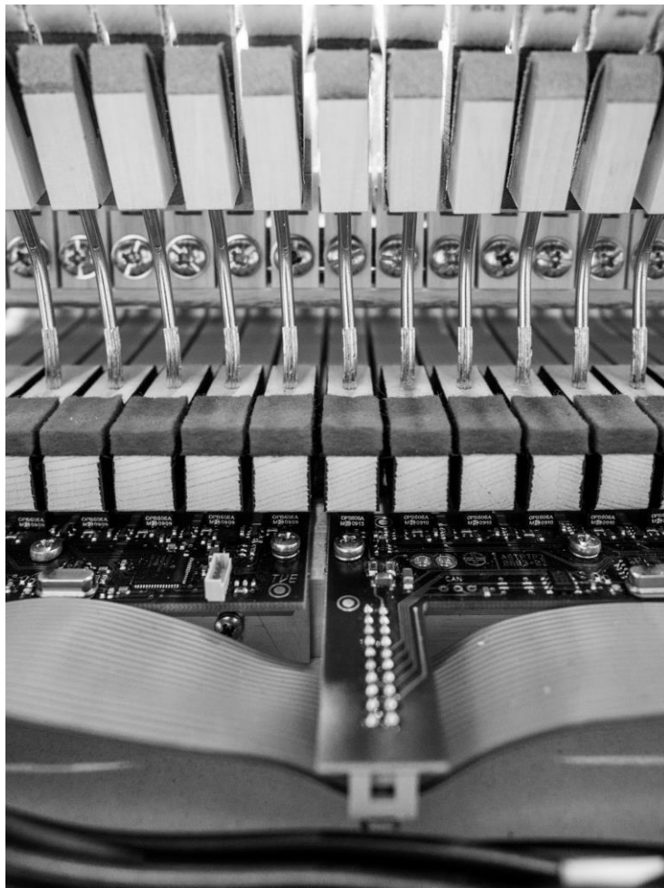
Detailaufnahme Mechanik + Elektronik Alpha Studio
